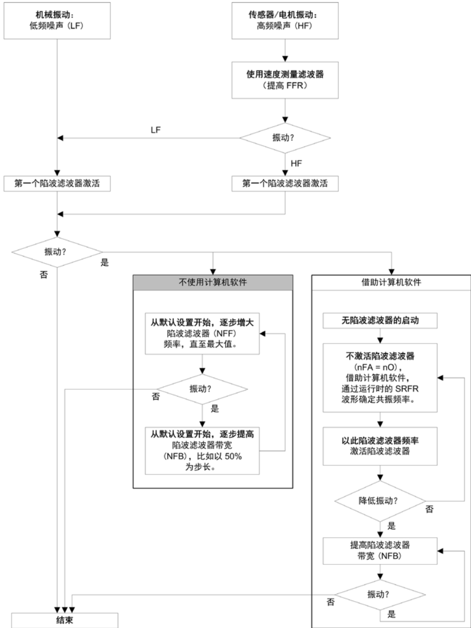
陷波滤波器设置
